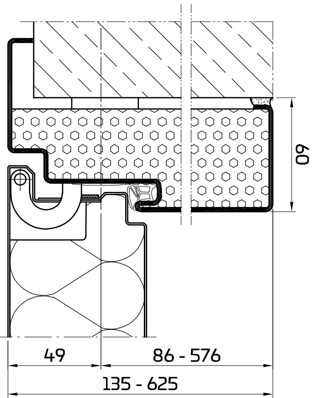
Umfassungszarge 00 / 30
