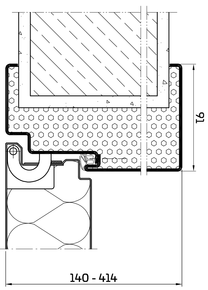
Zweiteilige Umfassungszarge 00 / 30
