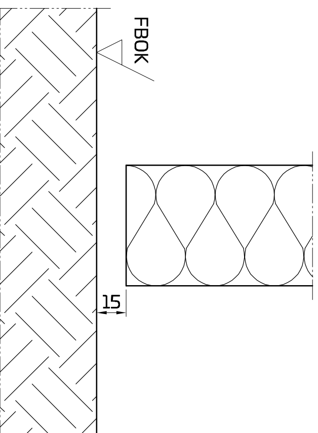
Bodenabschluss Bodenluft 15 mm
