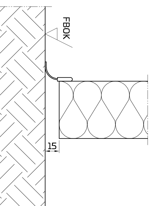
Bodenabschluss mit Rauchschutz
