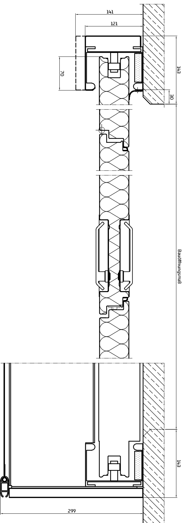
Horizontalschnitt Seitenführung Hubtor mit eingebauter Schlupfrühr
