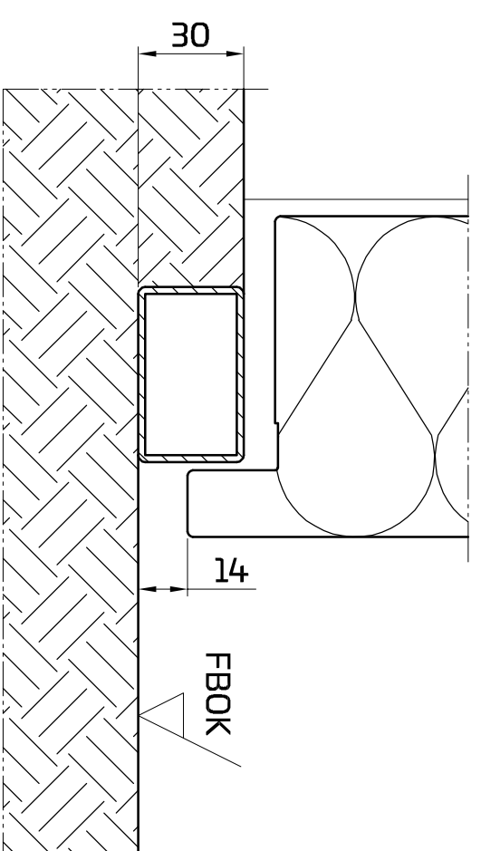
30 mm Formrohr + Türblatt vierseitig
