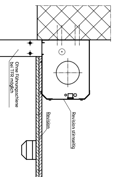
Wandmontage Gehäuse in der abgehängten Decke nicht sichtbar
