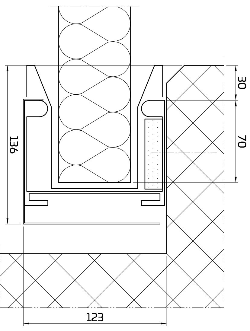
Normal einlaufend Betonwand
