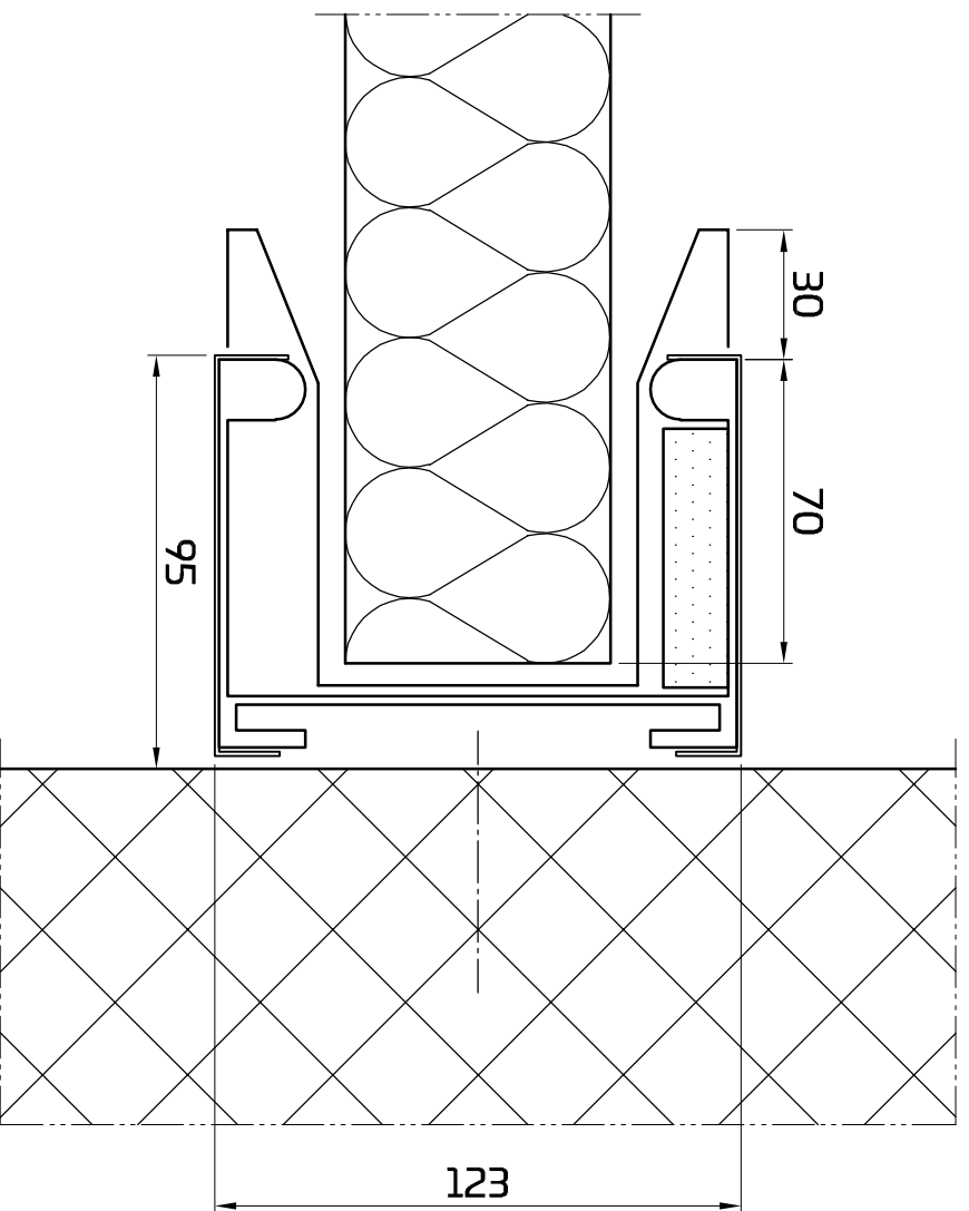
Stumpf einlaufend Betonwand
