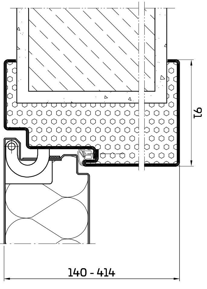
Zweiteilige Umfassungszarge 00 / 30
