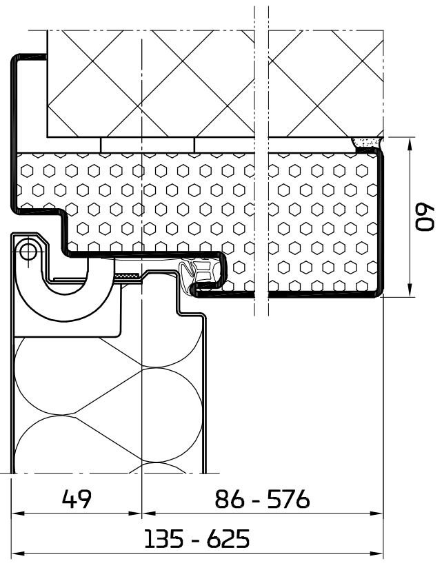
Umfassungszarge 00 / 30
