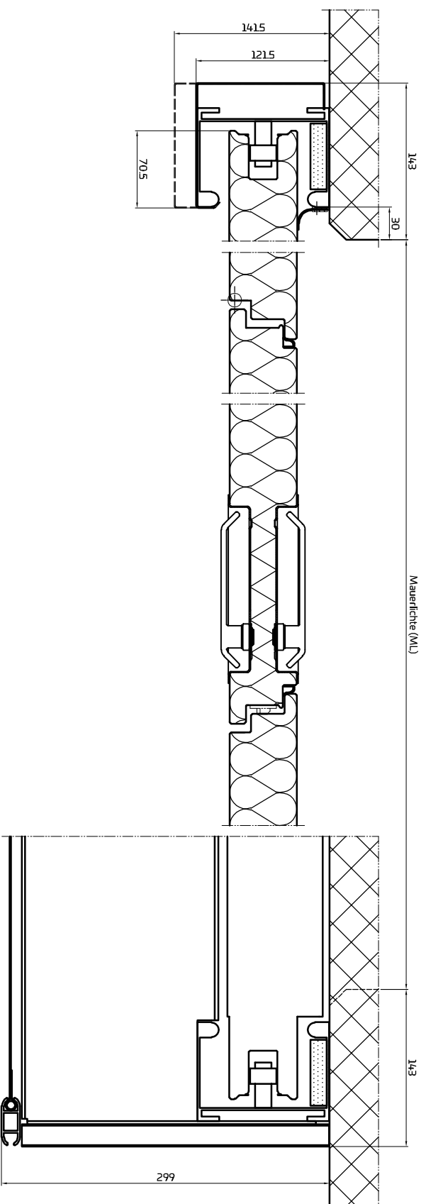
Seitenführung Hubtor mit Rauschutz und eingebauter Fluchtür (EFT)
