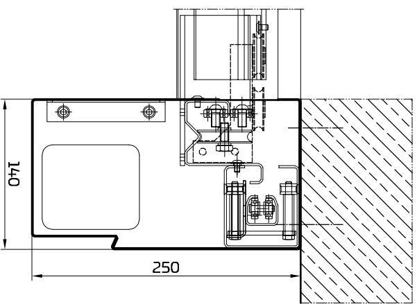
Seitliche Führung Deckenmontage
