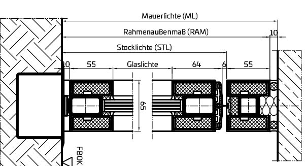
Mit Bodentürschleiber
