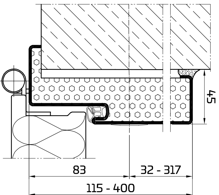
Umfassungszarge
