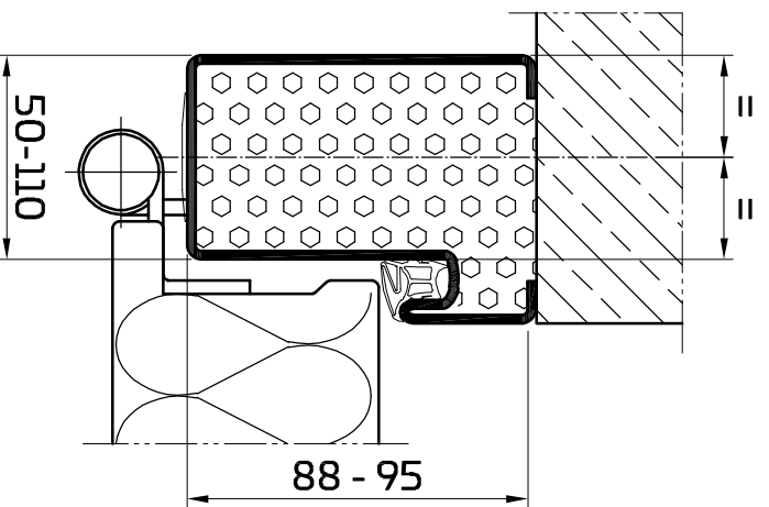
Vorsatzzarge variabel
