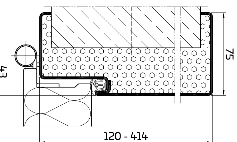
Umfassungszarge in DN geteilt
