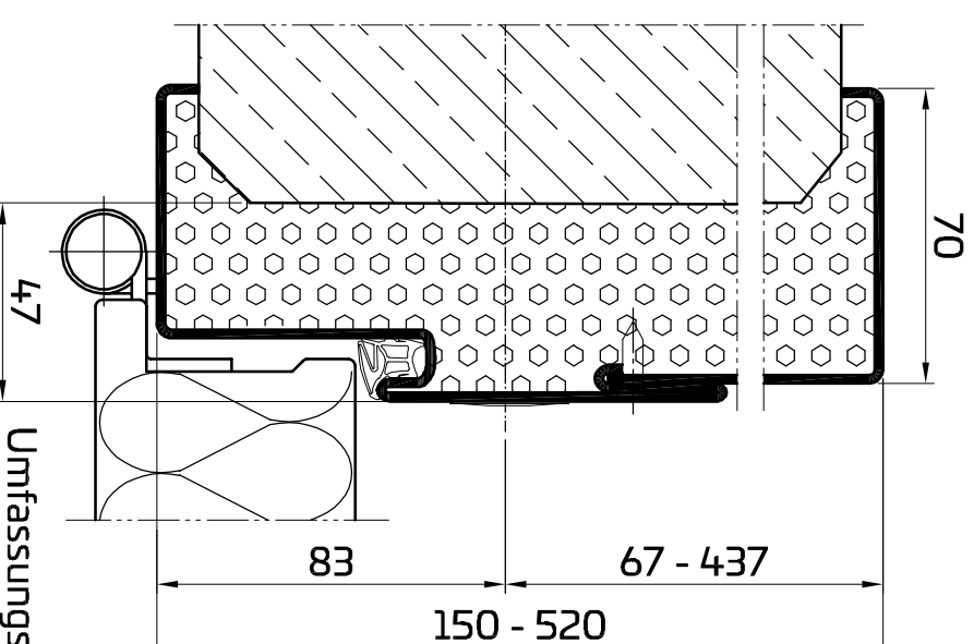
Umfassungszarge
