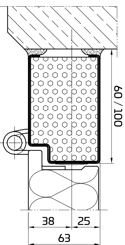
Stumpfzarge
