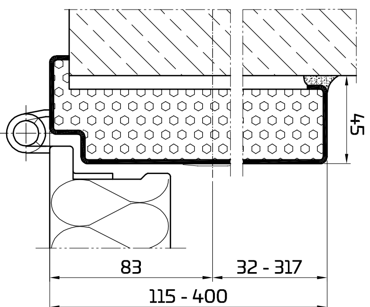
Umfassungszarge
