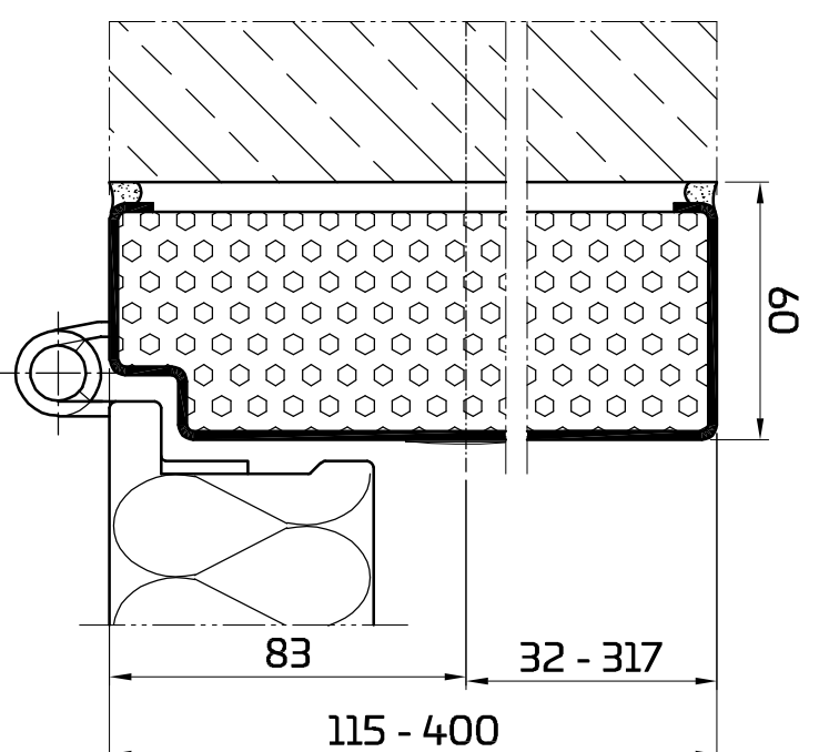
Umfassungszarge
