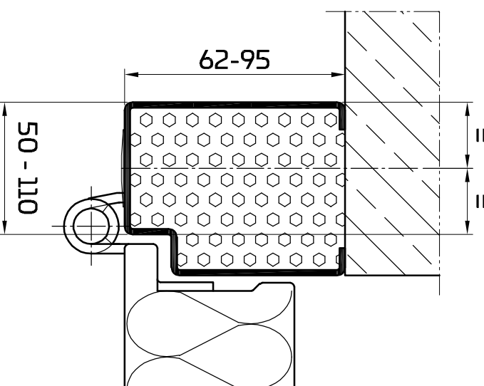
Vorsatzzarge variabel
