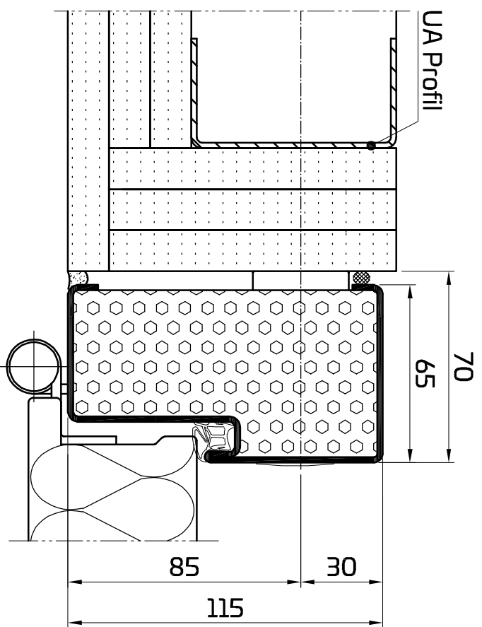
Blockzarge überfälzt mit Dichtnut 00 / EI30 Sa / S200
