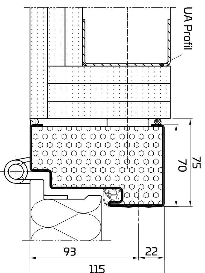
Blockzarge flächenbündig mit Dichtnut 00 / EI30 Sa / S200
