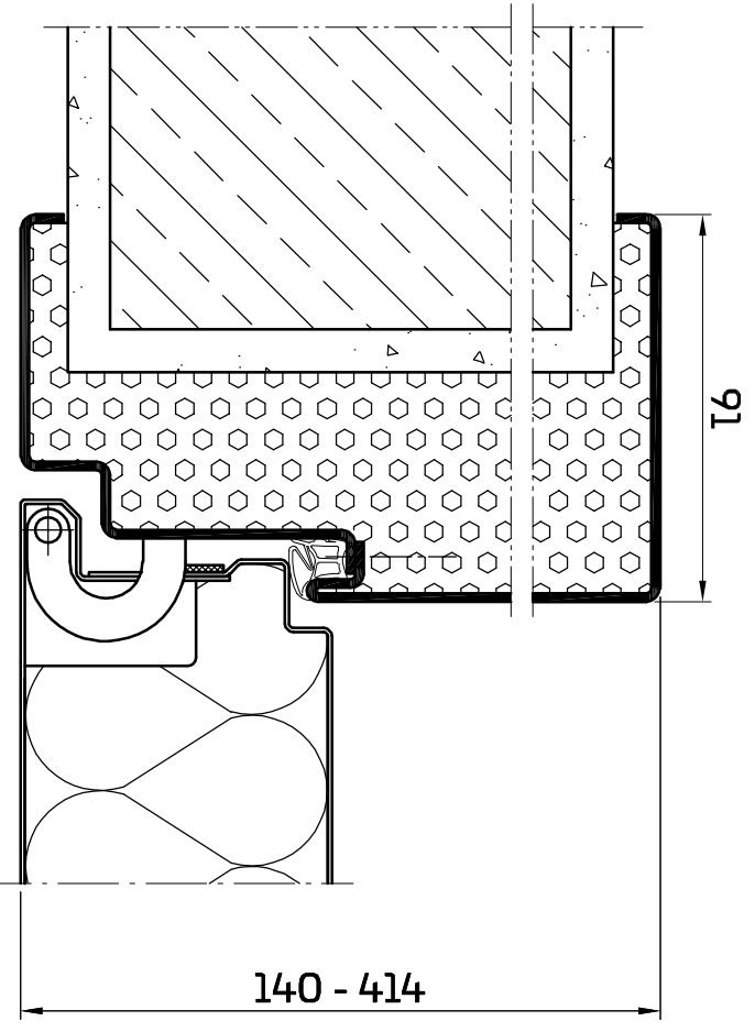
Zweiteilige Umfassungszarge 00 / 30
