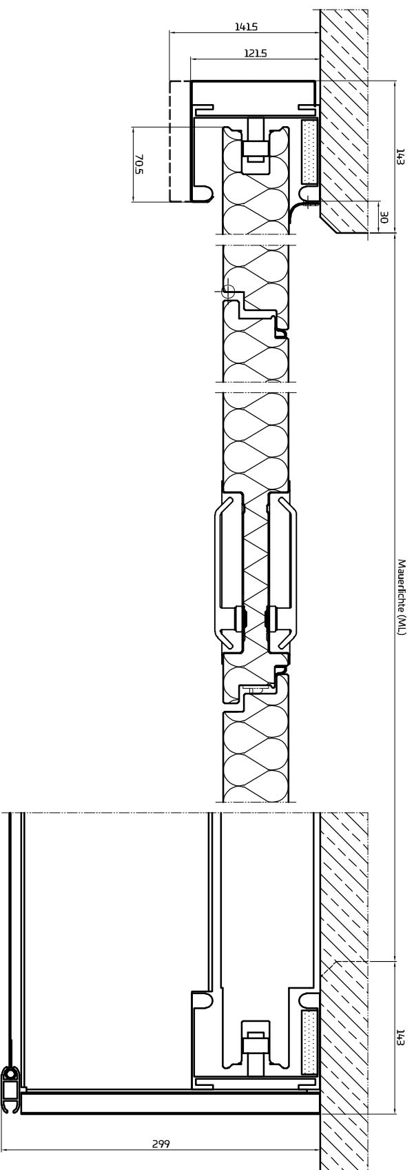
Seitenführung Hubtor mit Rauschutz und eingebauter Gehür
