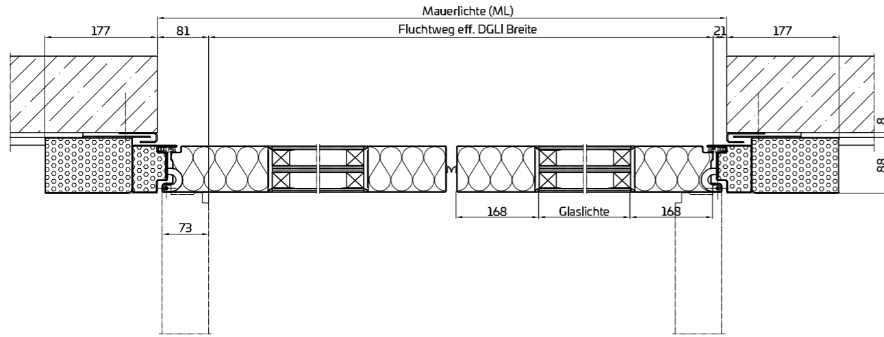
Horizontalschnitt aus der Laibung öffnend
