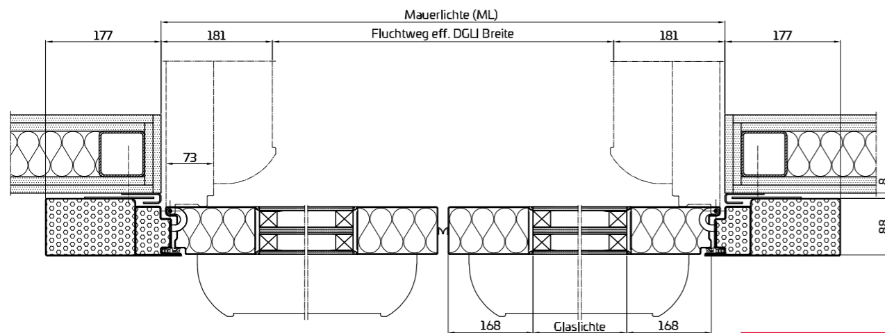
Horizontalschnitt in die Laibung öffnend * mit Beschlag
