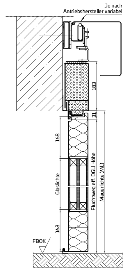
Vertikalschnitt aus der Laibung öffnend
