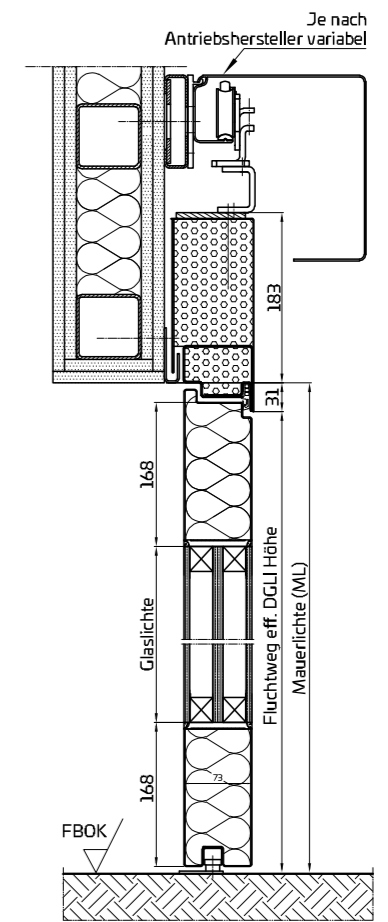
Vertikalschnitt in die Laibung öffnend
