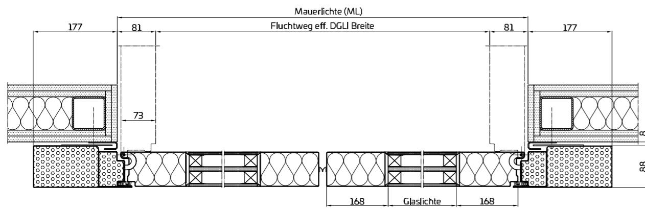
Horizontalschnitt in die Laibung öffnend *
